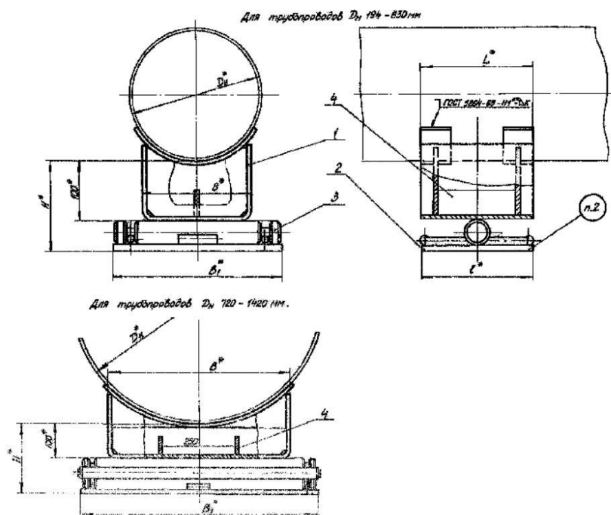
T19.00.00.000СБ – опора однокатковая
