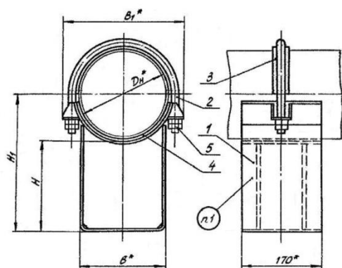
T16.00.00.000СБ – опора скользящая диэлектрическая
