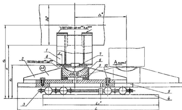
T21.00.00.000СБ – опора шариковая
