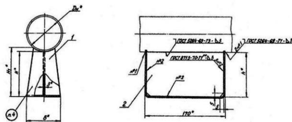
Т13.00.00.000СБ – опора скользящая
