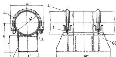
T18.00.00.000СБ – опора скользящая диэлектрическая
